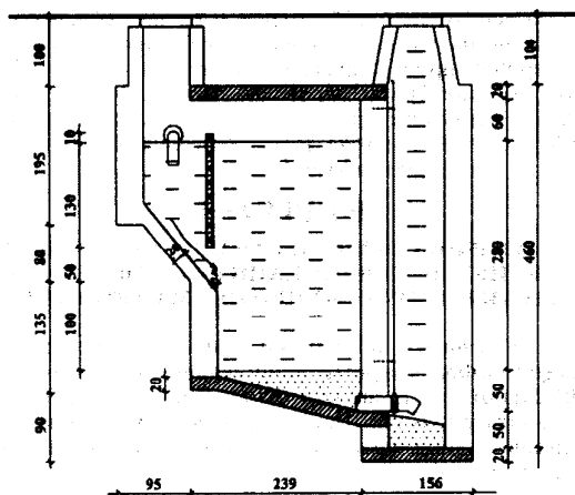
ТИП 2 - ЕМШЕРОВА ЈАМА ПРАВОУГАОНОГ ОБЛИКА
