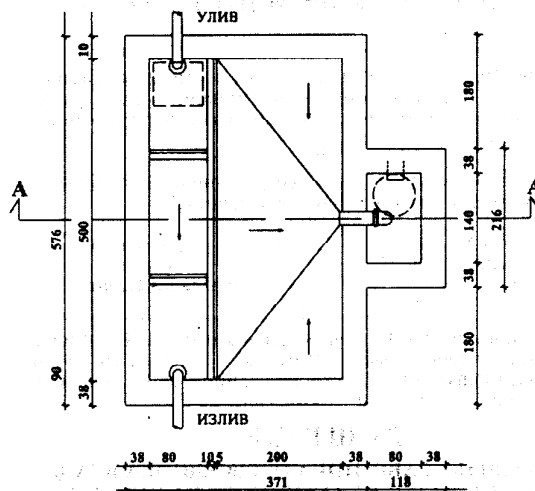
ТИП 2 - ЕМШЕРОВА ЈАМА ПРАВОУГАОНОГ ОБЛИКА
