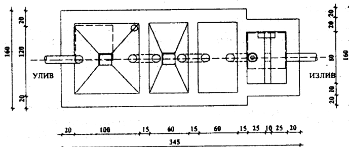
ТИП 1 - СЕПТИЧКА ЈАМА СА ТАЛОЖНИЦАМА И ДЕЗИНФЕКЦИЈОМ ПОМОЋУ ХЛОРИНАТОРА
